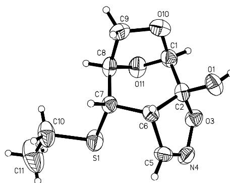
Fig. 2 ORTEP drawing of (1 R ,2 R ,6 S ,7 S ,8 R )-7-Ethylthio-4-aza-3,10,11-trioxa-tricyclo[6.2.1.0 2,6 ]undec-4-en-2-ol ( 8 )
